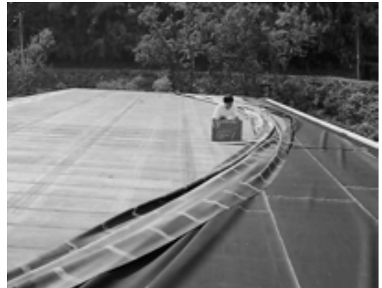
▲防水シートのはがれた立小野小体育館屋上
