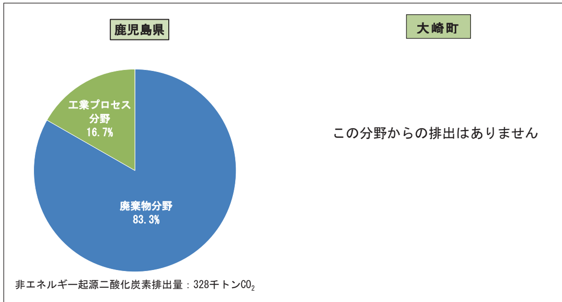
2019年度の非エネルギー起源二酸化炭素排出割合 資料 鹿児島県：県温暖化対策実行計画改定にかかるパブコメ資料
