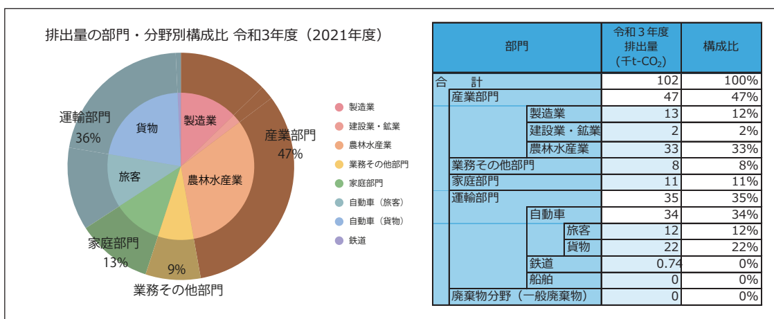
排出量の部門・分野別構成比 2021（令和3）年度
